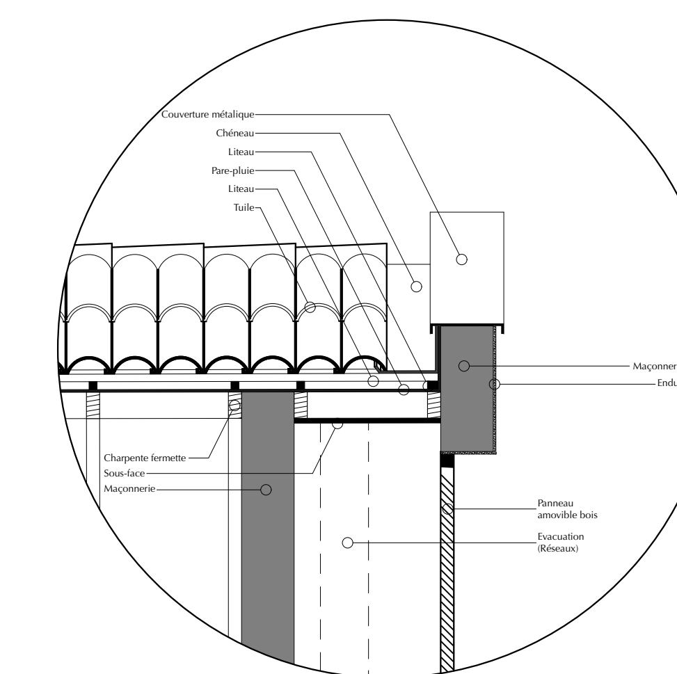
Détail 1 - Ech: 1/20
