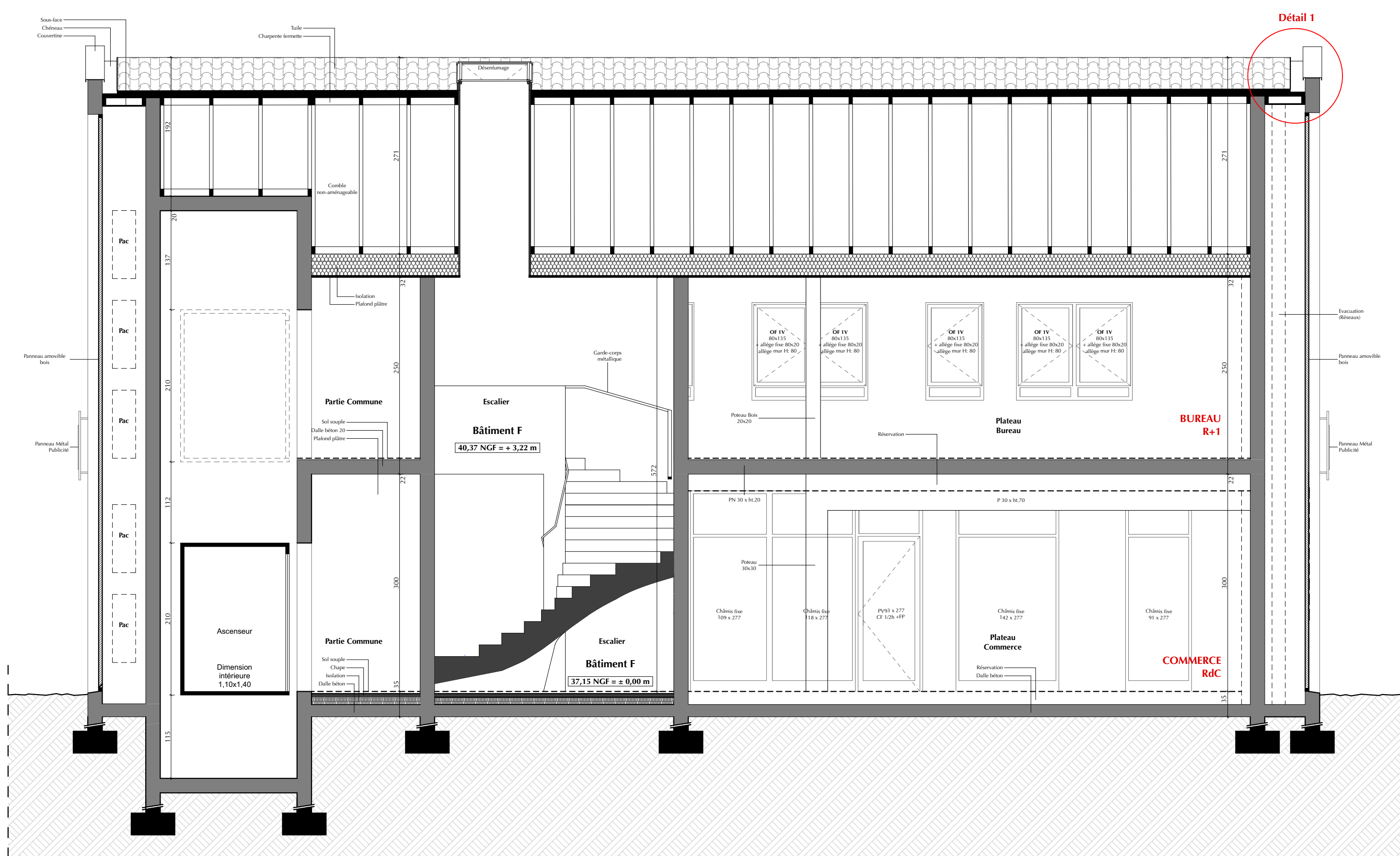
Coupe AA' - Ech: 1/50
